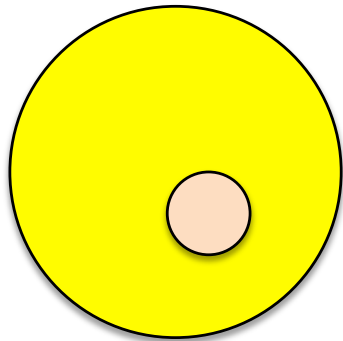
a) Binaria eclipsante de baja masa
