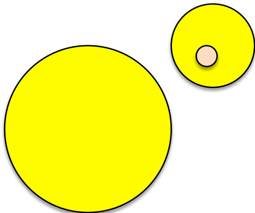
d) Binaria eclipsante de fondo
