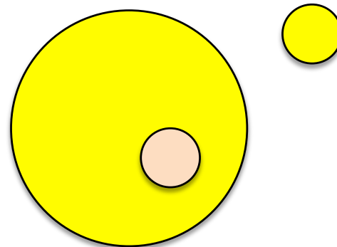
b) Binaria eclipsante de baja masa + estrella de fondo
