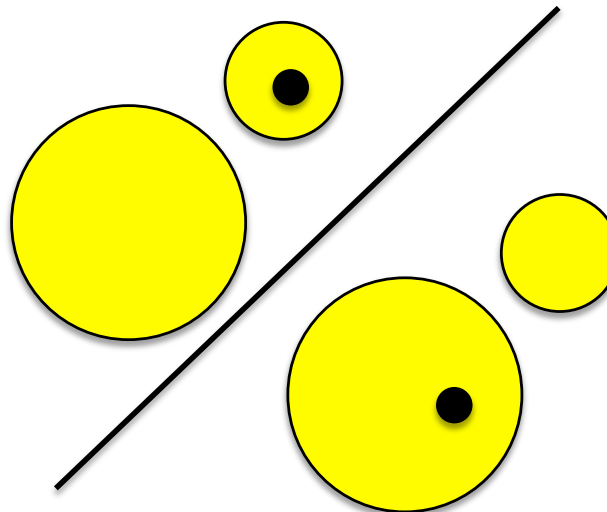
e) Planetas más grandes ocultos por estrellas de fondo
