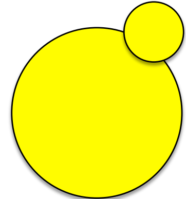
c) Tránsito parcial de una binaria eclipsante
